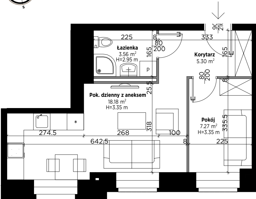
RZUT KONDYGNACJI SEGMENT A
