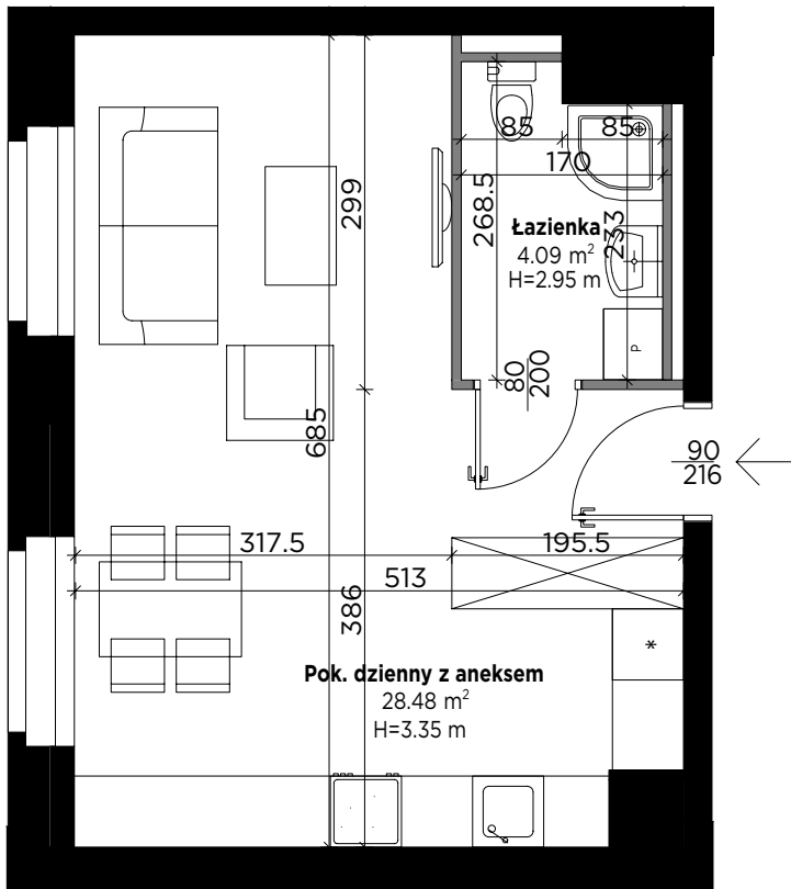
RZUT KONDYGNACJI SEGMENT A
