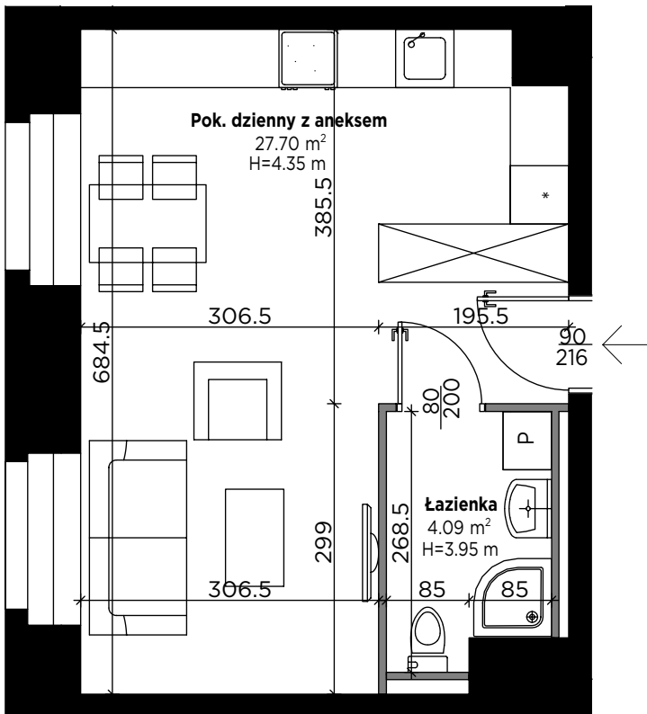
RZUT KONDYGNACJI SEGMENT A
